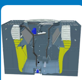
Esecuzione per alte temperature CPVC BACross 2 pacco di scambio
